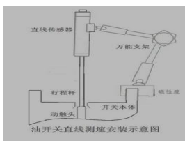
油开关直线测速安装示意图
