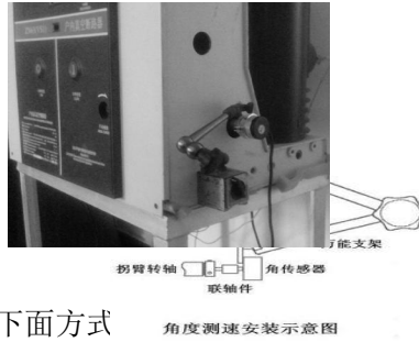
角度测速安装示意图
